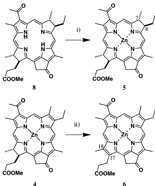
Scheme 2. i) \text{Zn}(\text{OAc})_2 \cdot 2\text{H}_2\text{O} / \text{MeOH}-\text{CH}_2\text{Cl}_2 ; ii) DDQ/ \text{CH}_3\text{COCH}_3 .
